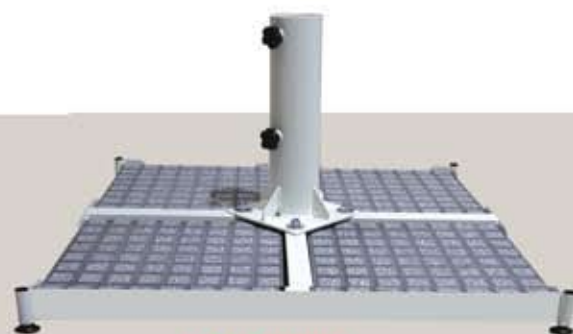
Art. A 1090-60 βάση μεταλλική μεταφερόμενη για 4 πλάκες πεζοδρομίου 40x40 cm, για ιστό Φ 60-90mm, συνολικό μέγεθος 88x88 cm
